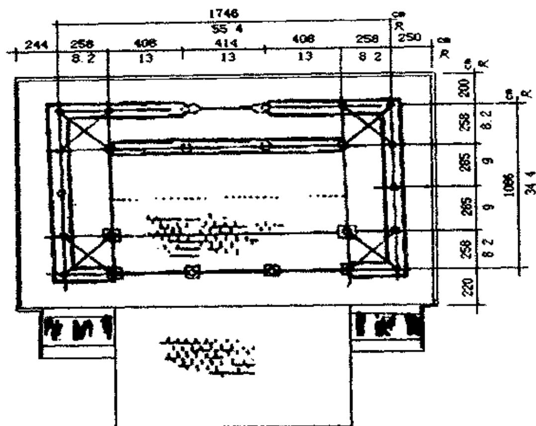
永济永乐宫重阳殿平面图
