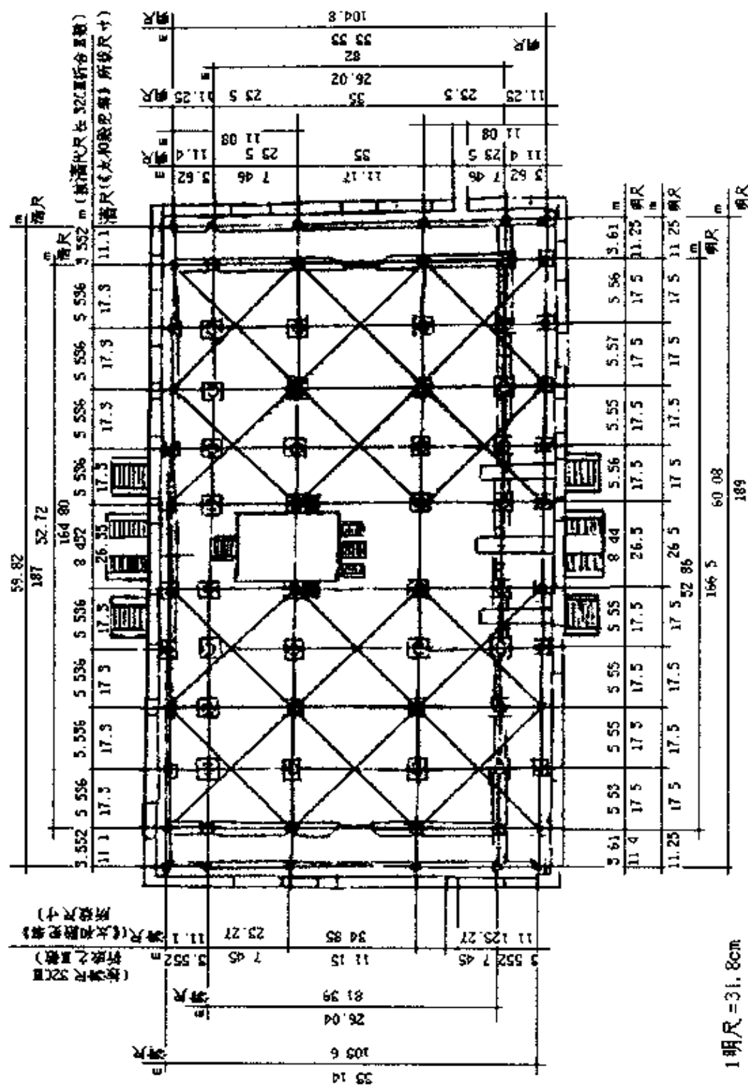
北京紫禁城太和殿平面图
