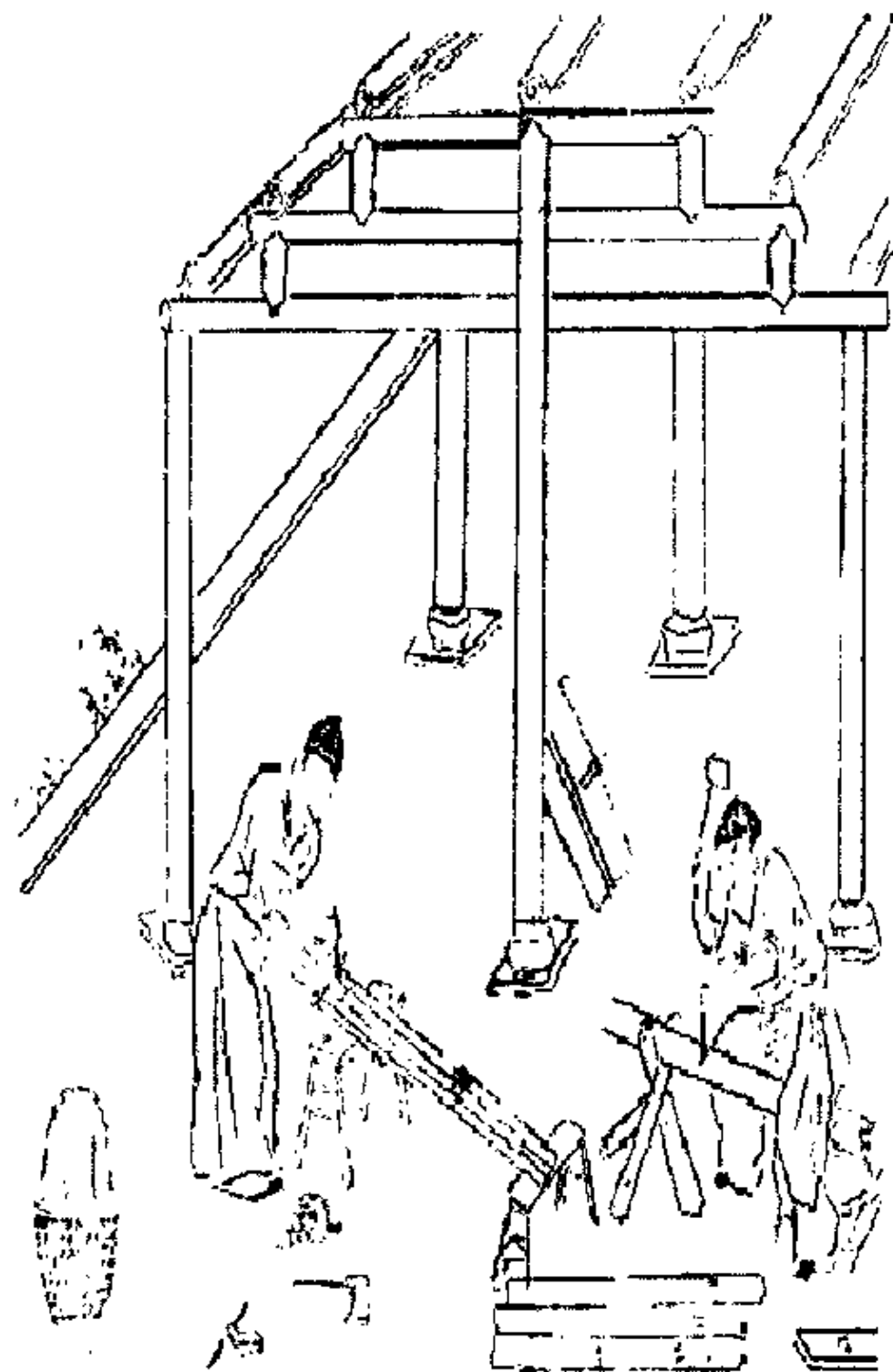
正七架格式(原图)
