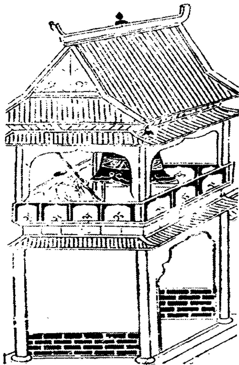
建钟楼格式(原图)
