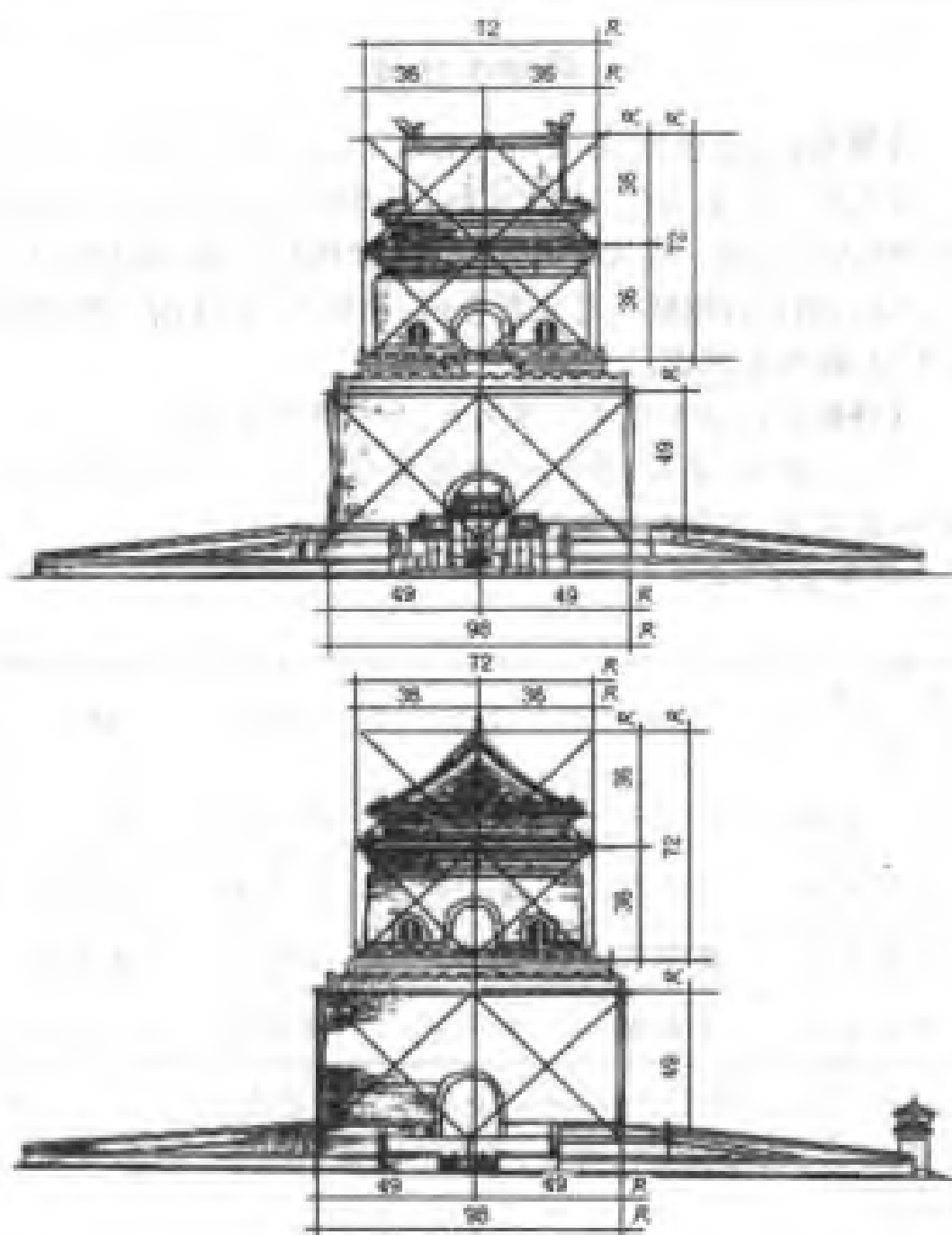
北京钟楼正立面及侧立面图
